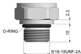
9/16-18UNF-2A
