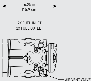
700 Series 12 Volt Top
