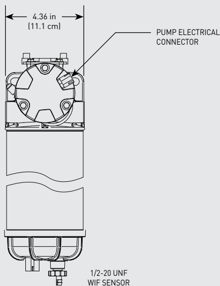
700 Series 12 Volt Front
