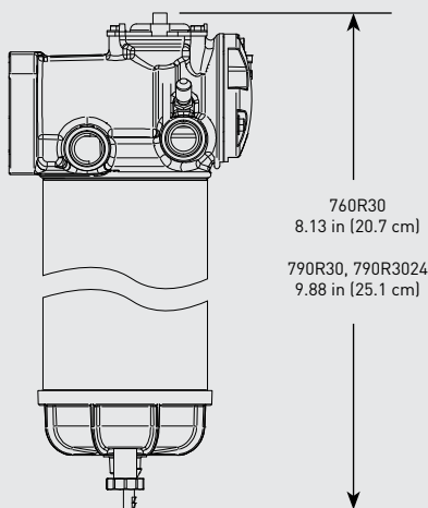
700 Series 12 Volt Profile
