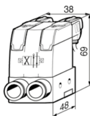
Ventilmodul Größe 2
