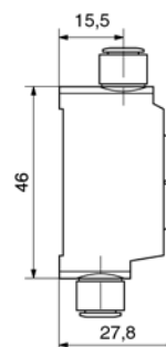
Drehbarer Steckanschluss für 4 mm AD Rohr
