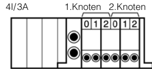
AS-i Ausf. 2 - 1 Knoten Modul
