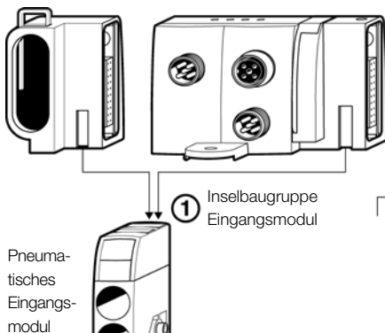
Elektro-Eingangsmodul der Ventilinsel: Mehrfachstecker oder Feldbusanschluss
