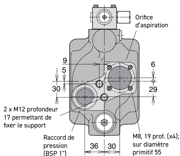
Vue A-A
