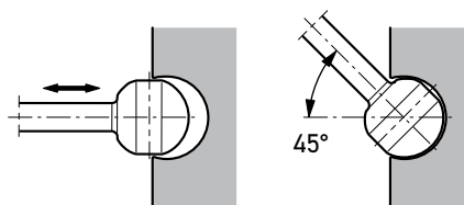
Verrouillage de piston dans l'arbre F3
