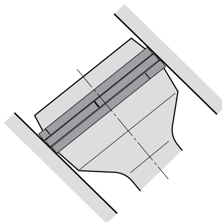
F1 piston avec segment lamellaire
