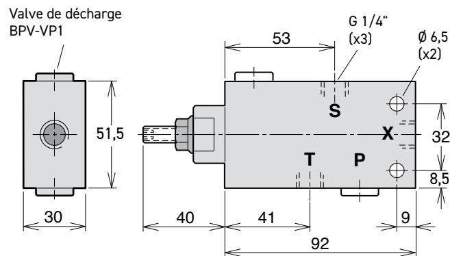
Valve de décharge BPV-VP1
