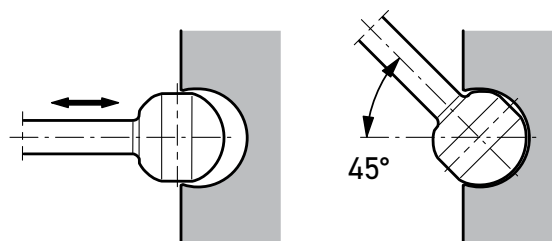
Verrouillage de piston dans l'arbre F1
