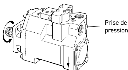
Fig. 5. Pompe à rotation à droite
