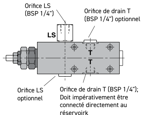
Régulateur (VP1-095/-110/-130).
