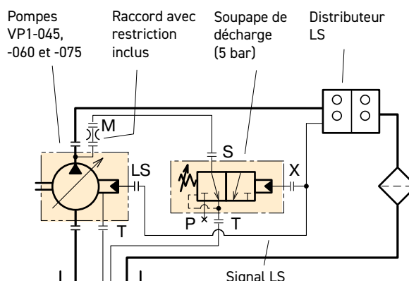
Schéma Hydraulique de BPV-VP1 pour les pompes VP1-045, -060 ou -075.
