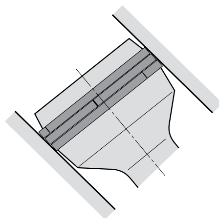
F3 piston avec segment lamellaire
