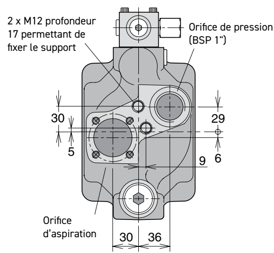
Vue A-A
