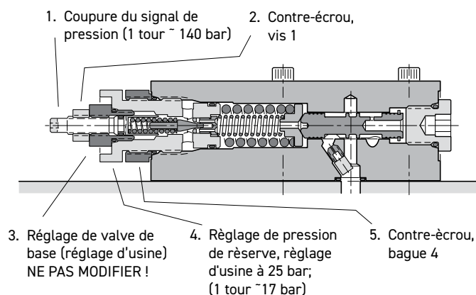
Vue en coupe de la commande LS.
