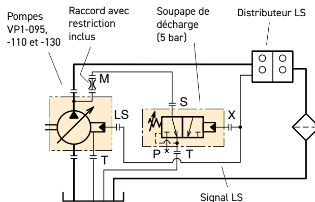
Schéma Hydraulique de BPV-VP1 pour les pompes VP1-095, -110 ou -130.
