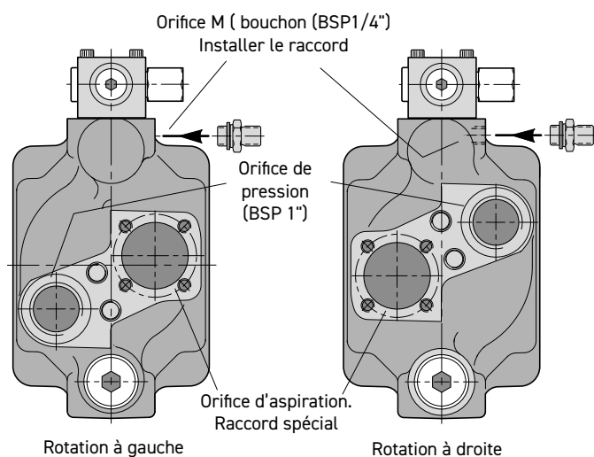
(VP1-095/-110/-130) Orifices principaux
