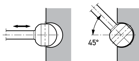
Verrouillage de piston dans l'arbre F4
