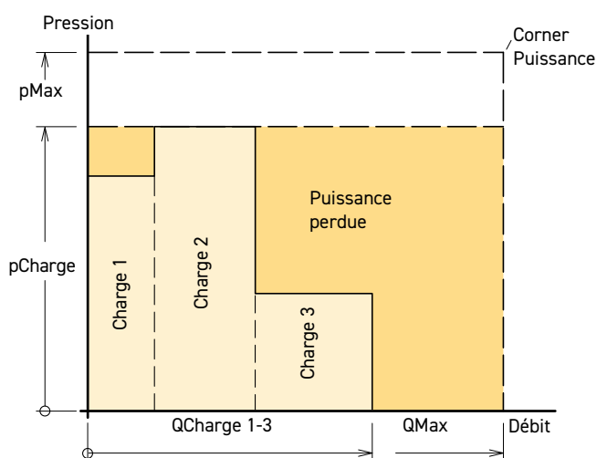
Diagramme 1. Système à débit constant: pompe à cylindrée fixe
