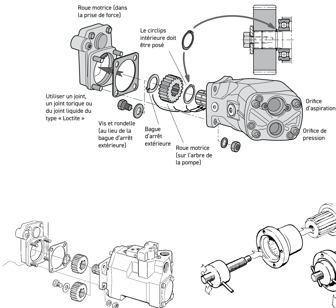
Fig. 6. Installation d'une pompe sur une prise de force
