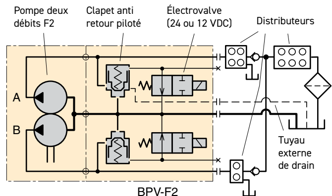
Schéma hydraulique ( système avec valve de décharge ; exemple )
