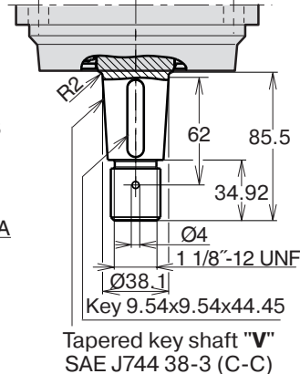
Shaft option V (F10-56)
