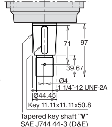
Shaft option V (F10-80)
