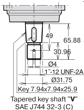
Shaft option V (F10-30, F10-37)
