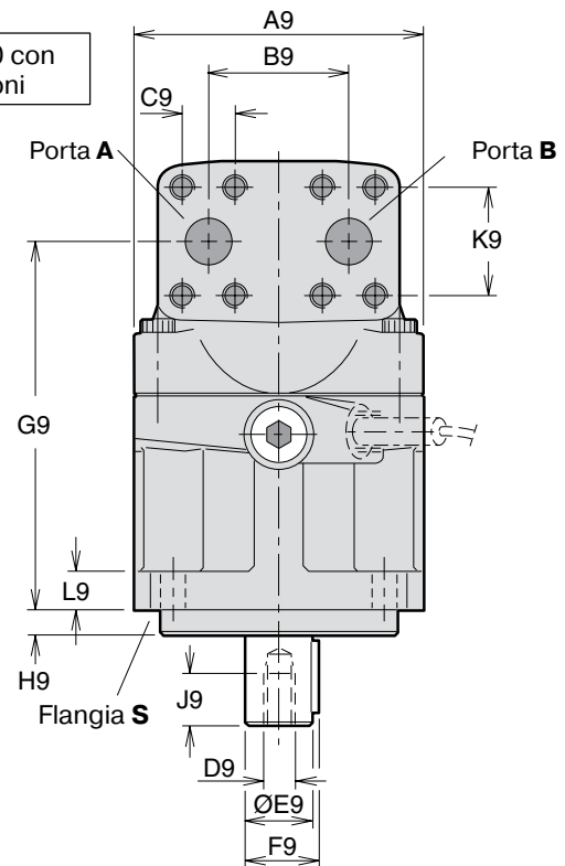
Porta E (drenaggio) F12-110 e -125 alloggiamento corpo cilindri (versione SAE)
