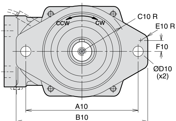
Flangia di montaggio tipo T (SAE 2 bulloni)
