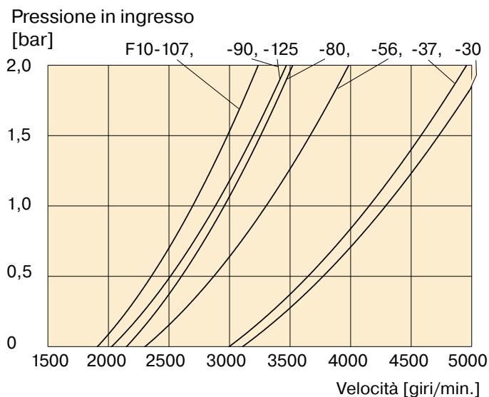
Diagram 2 Pressione in ingresso min richiesta (F10-L o R)
