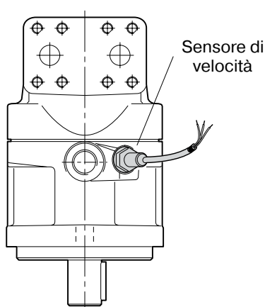
F10/F12 con sensore di velocità.
