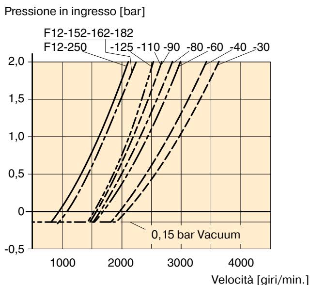
Diagramm 3. Pressione in ingresso min richiesta motore (F12-M).
