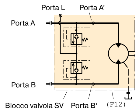
Schema idraulico
