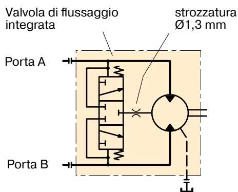
Schema idraulico.
