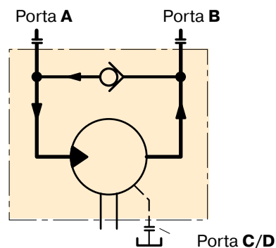
Schema del motore per ventole con valvola anticavitazione
