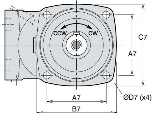
Flangia di montaggio tipo S (SAE, 4-Loch)
