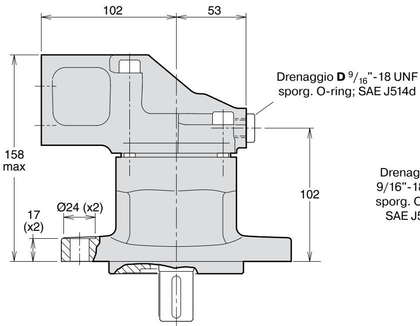
Porta principale A 1 1/16" - 12 UN sporg. O-ring; SAE J514d
