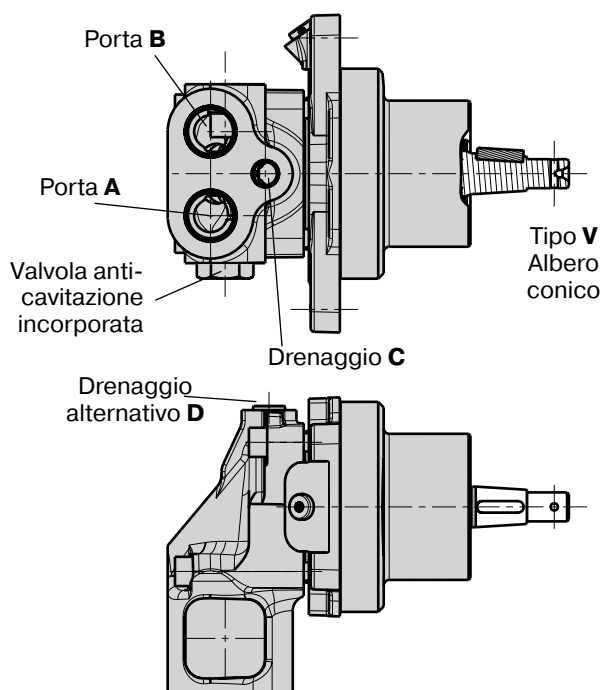
Motore per ventola (F11-10 in figura).
