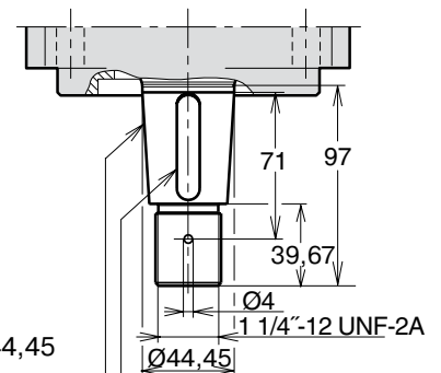
Albero conico con chiavetta "V" SAE J744 44-3 (D&E)
