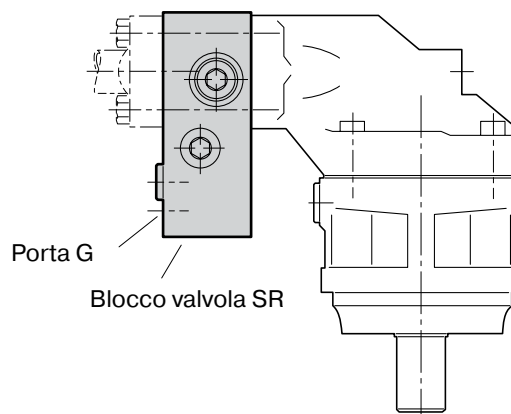
Posizione del blocco valvola SR
