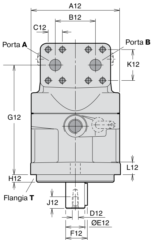
In figura: F12-60 con flangia 2 bulloni
