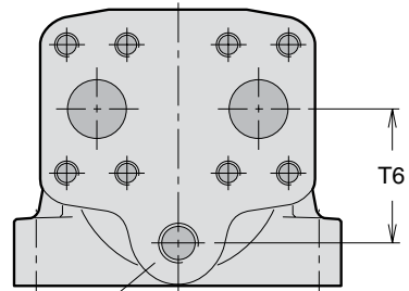
Porta E (drenaggio) F10-125 alloggiamento corpo cilindri (versione ISO / cartuccia)
