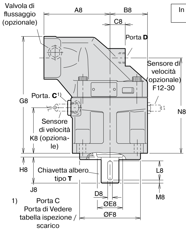
Flangia di montaggio tipo S (SAE, 4-Loch)
