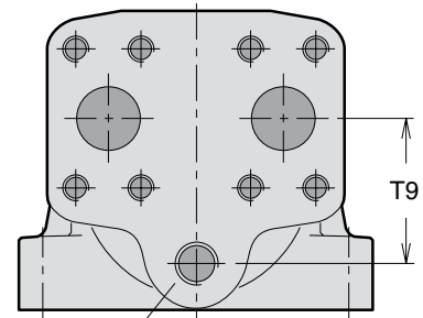
Porta E (drenaggio) F12-110 e -125 alloggiamento corpo cilindri (versione SAE)
