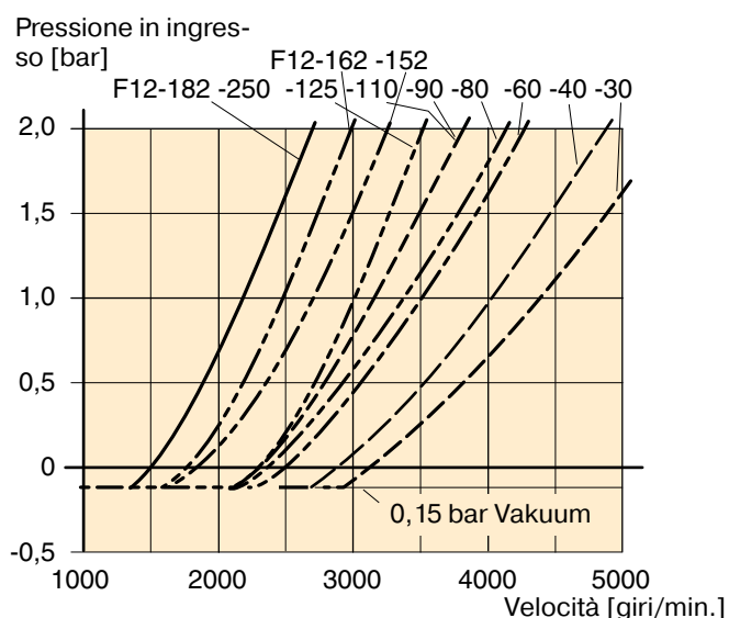
Diagramm 2. Pressione in ingresso min richiesta pompa (F12-L o -R).
