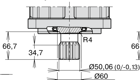
Albero scanalato tipo F SAE J498b, classe 1; 15T-8/16 DP; filettato, lato piatto
