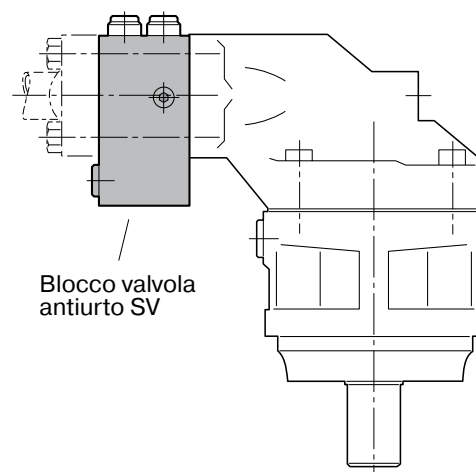
Blocco valvola SV installato su un motore F12
