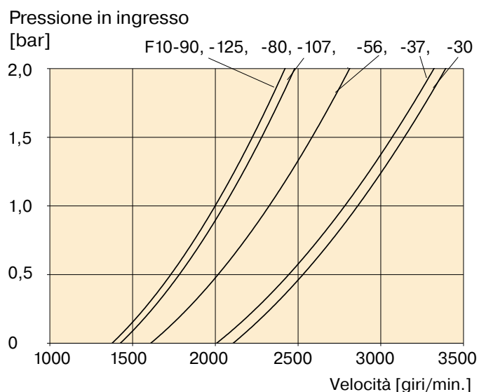
Diagram 3 Pressione in ingresso min richiesta (F10-A)
