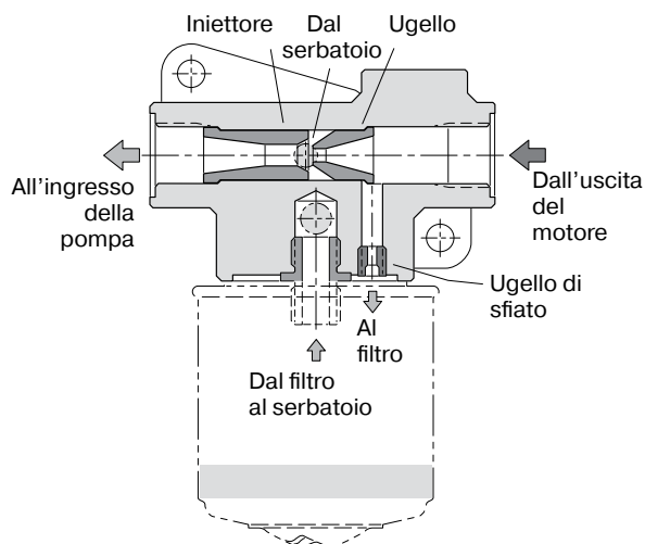
Sezione del booster BLA.
