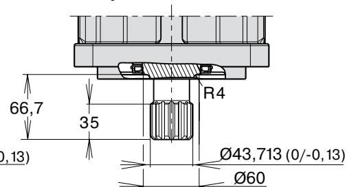
Albero scanalato tipo S SAE J498b, classe 1; scan. involuta 30°; 13T-8/16 DP; lato piatto
