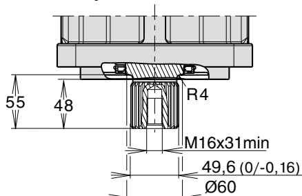
Scanalatura albero tipo D W50x2x24x9g DIN 5480
