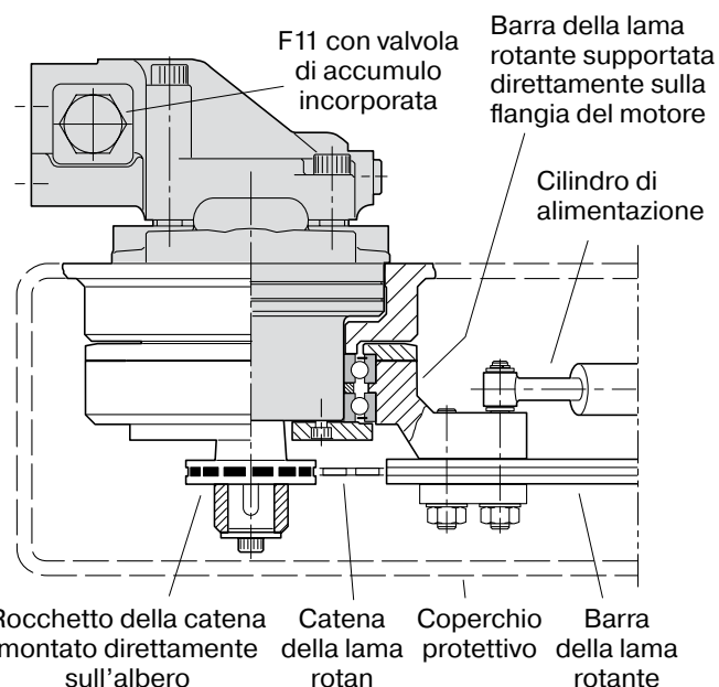
Esempio di installazione della lama rotante catena (F11-10 in figura)
