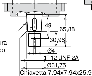
Albero conico con chiavetta "V" SAE J744 32-3 (C)
