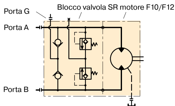
Schema del blocco valvola SR.
