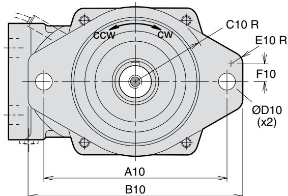
Flangia di montaggio tipo T (SAE 2 bulloni)
