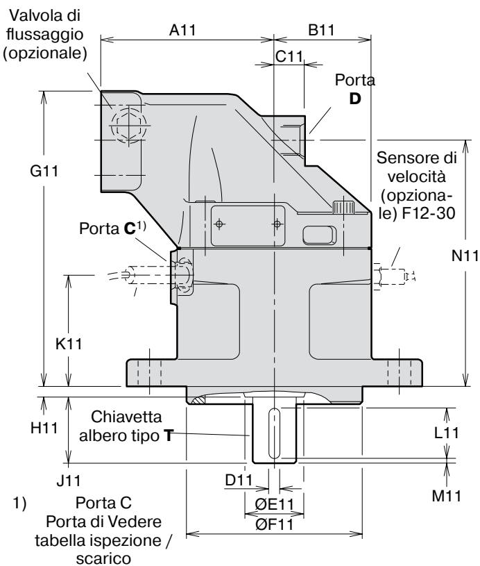
Flangia di montaggio tipo T (SAE 2 bulloni)
