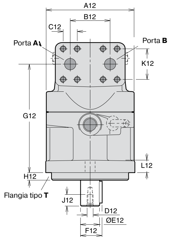
Abb. F10-80 mit 2-Loch Flansch
