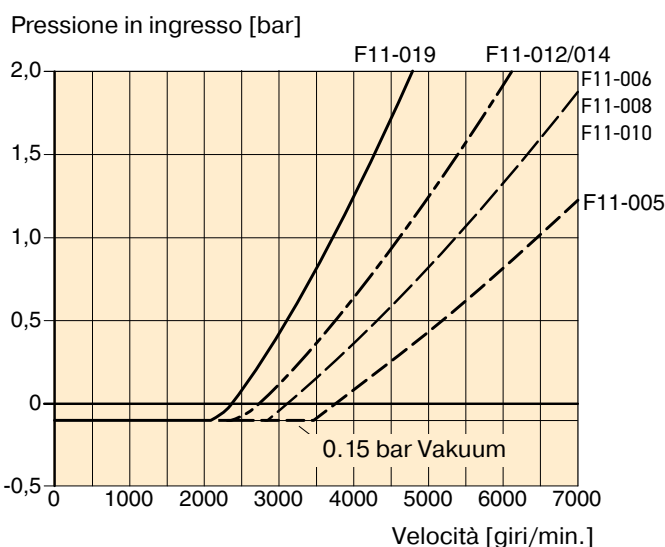
Diagramm 1. Pressione in ingresso min richiesta
