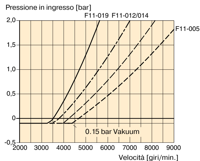
Diagramm 2. Pressione in ingresso min richiesta
