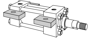
Centerline Lug Model 73 (NFPA MS3)
