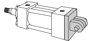
Detachable Clevis Model 86 (NFPA MP2)
