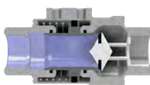
Position vanne axiale fermée
