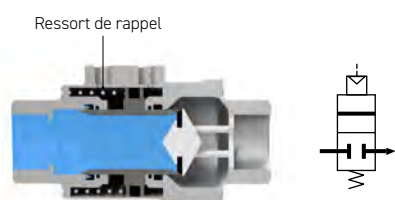
État repos (vanne fermée)
