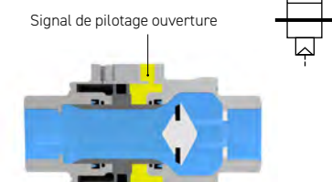
État piloté (vanne ouverte)
