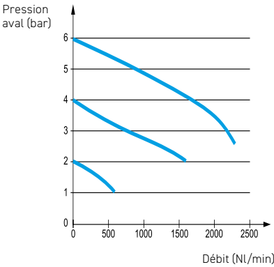
Modèles G3/8
