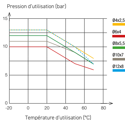
Tube polyuréthane anti-étincelles (monocouche)
