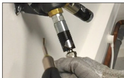
Facilité d'utilisation grâce au bouton poussoir qui active la purge
