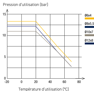
Tube polyuréthane anti-étincelles, avec gaine PVC
