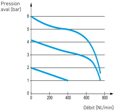
Modèles G1/8
