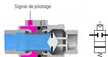
État piloté (vanne fermée)
