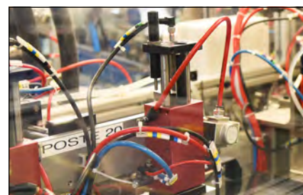
Assemblage pneumatique dans un environnement industriel restreint
