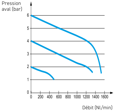
Modèles G1/4
