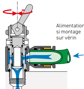
Levier orientable
