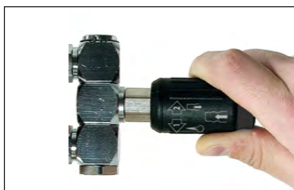
Purge activée par rotation de la bague
