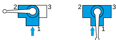
Passage à gauche
