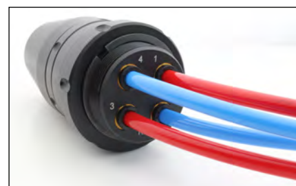
Multi-connecteur cylindrique à monter sur une cloison dans un équipement industriel
