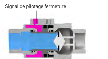
État piloté (vanne fermée)
