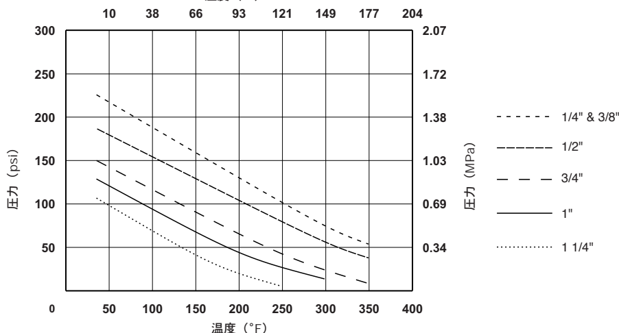
温度-圧力特性 温度 (°C)
