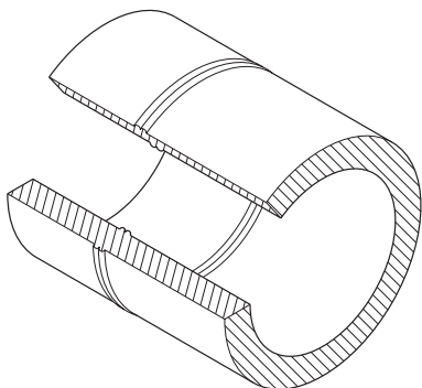
正しい接合
