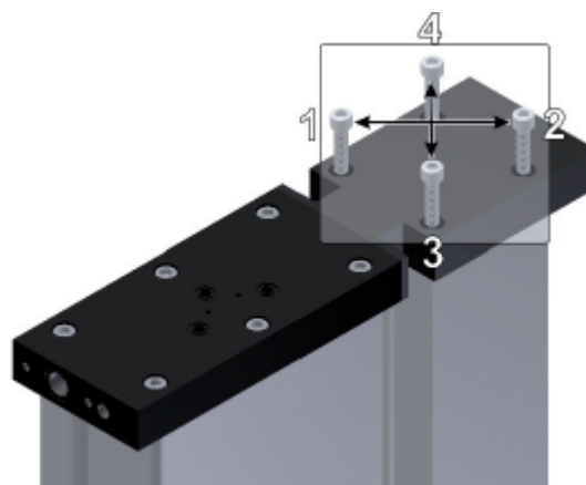
Prawidłowo zamocować płytę czołową
