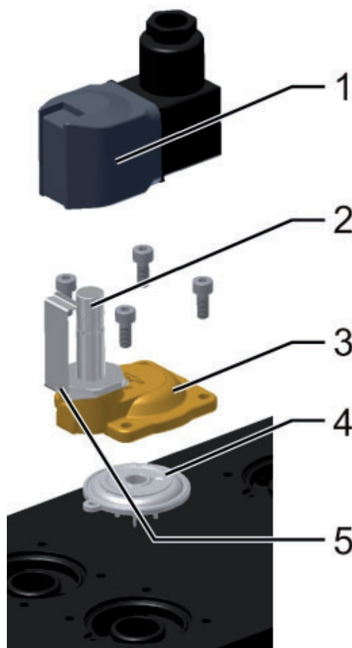
Zawór elektromagnetyczny
