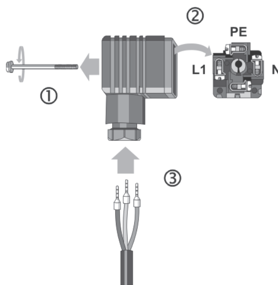
Conectar línea de alimentación eléctrica a la clavija de aparato
