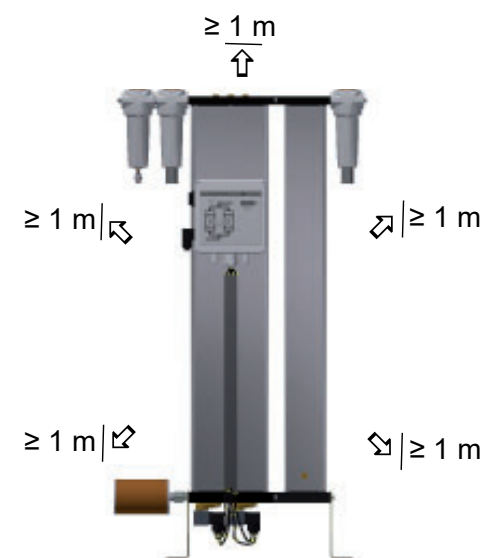
Distancia requerida hacia arriba y a los lados = mín. 1 m
