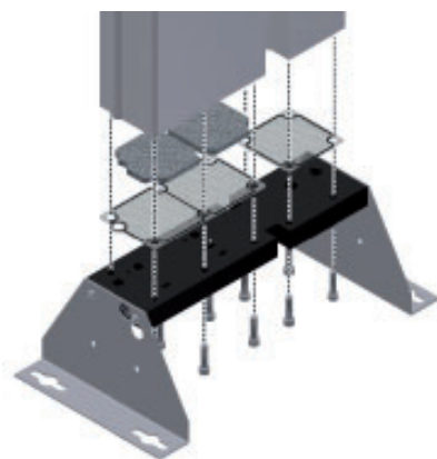
Aflojar placa de válvulas magnéticas
