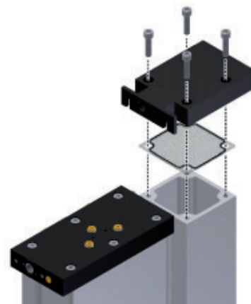
Aflojar placa superior
