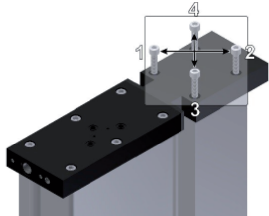
Fijar correctamente la placa superior
