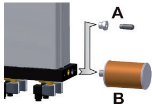
Aflojar el silenciador
