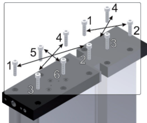
Fijar correctamente la placa de válvulas de retención
