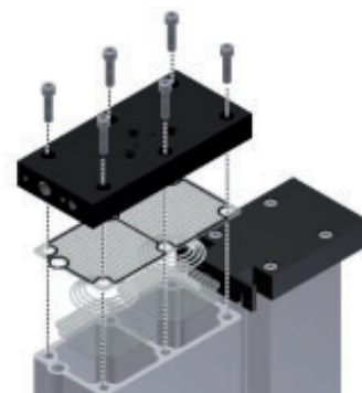
Aflojar la placa de válvulas de retención
