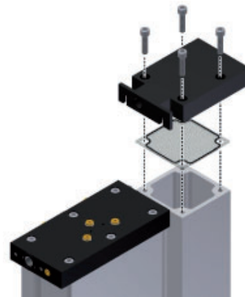
Kopfplatte lösen
