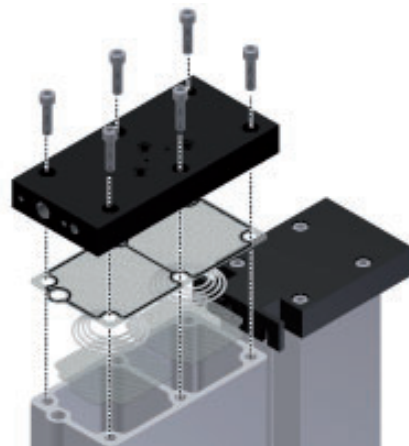
Rückschlagventilplatte lösen
