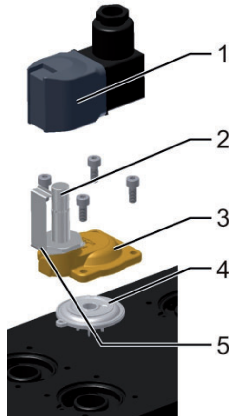
Magnetventil
