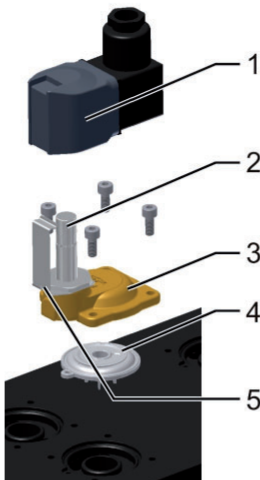
Solenoidový ventil
