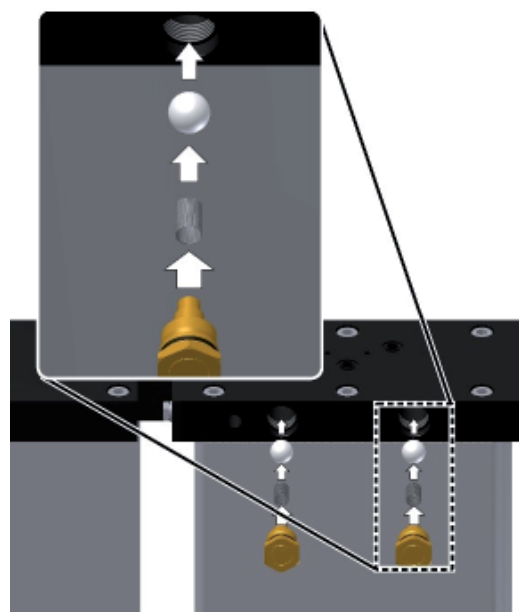
Zawory zwrotne
