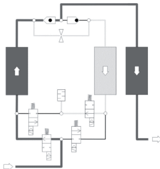
Adsorpcja w lewej komórce z granulatami osuszacza
