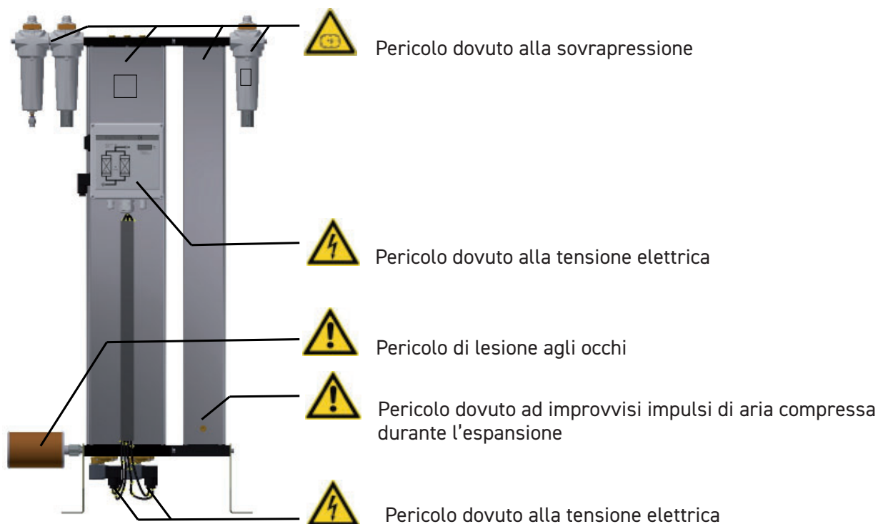
Vista anteriore
