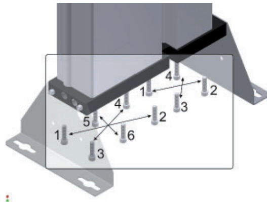
Fixer la plaque de l'électrovanne
