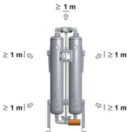
Distance nécessaire vers le haut et sur les côtés = min. 1 m
