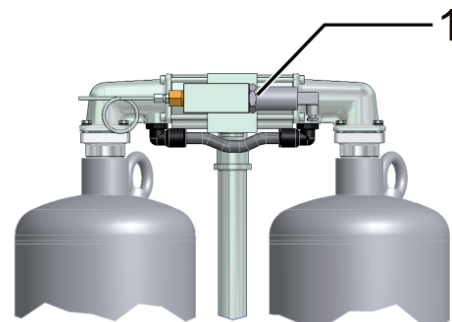
Capteur de point de rosée sous pression (1)
