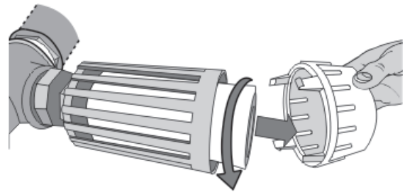
Cambiar el elemento del silenciador
