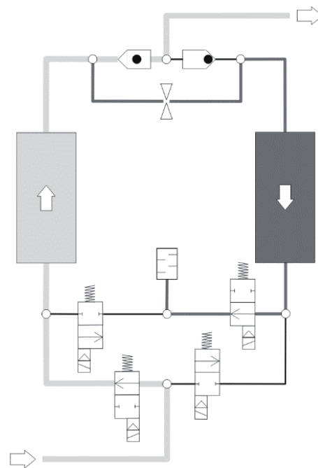
Regeneración en la cámara derecha
