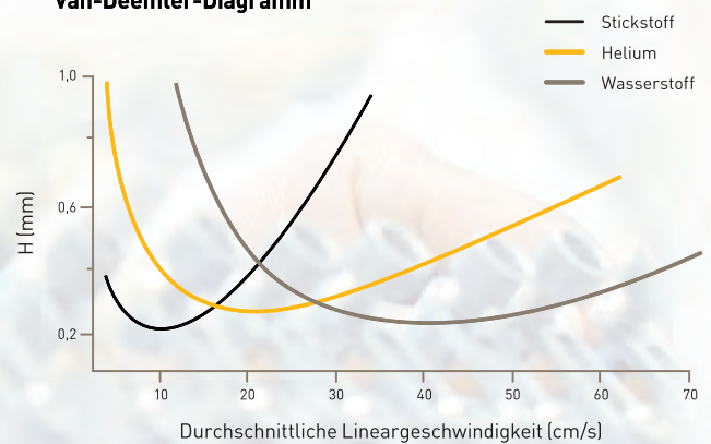
Van-Deemter-Diagramm
