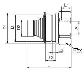
Tarudage Fourni avec circlips suivant DIN 471
