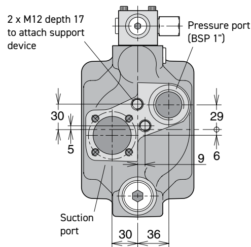
View A-A
