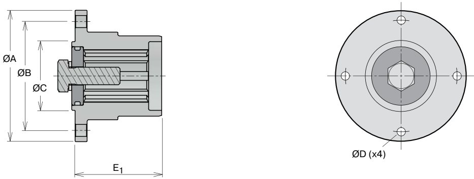
Fig. 2. DIN 90 (370 7423)
