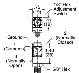
DIN Connector
