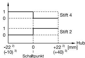
0: Spannung max. 1,8 V 1: Spannung min. U B =2,5 V
